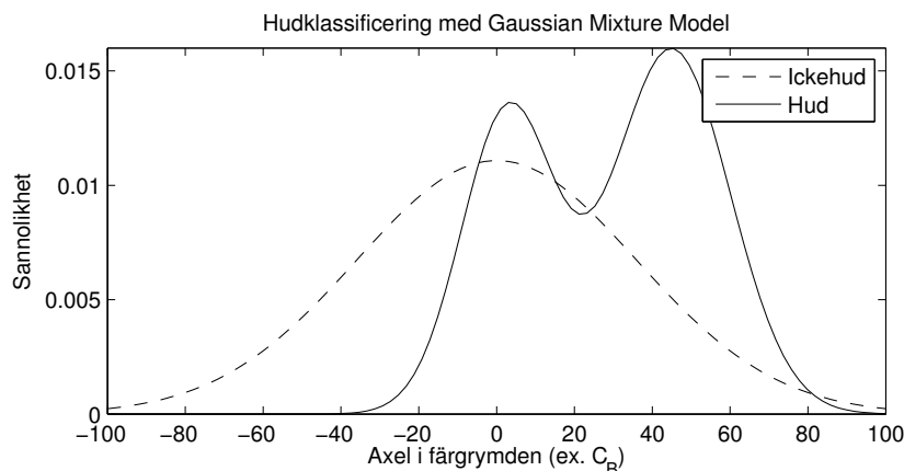
Figur 2.2: Ett exempel på hur sannolikhetsfördelningarna för hudfärg och ickehudfärg kan se ut längs en linje i C_b C_r -planet. Hudfördelningen är en linjärkombination av två normalfördelningar, medan ickehudfördelningen är en enkel normalfördelning. Exemplet är rent illustrativt, och bygger inte på resultat.
